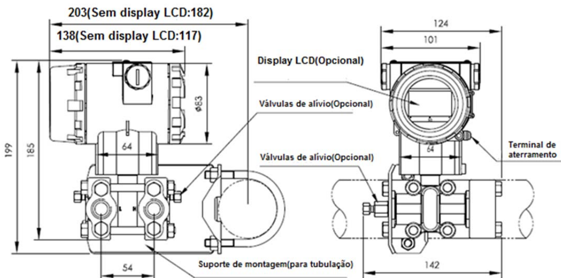
Tubulação montado na horizontal ( Vista lateral )
